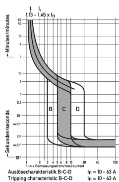
Diagramme Leitungsschutzschalter DLS 6hsl C10-1
