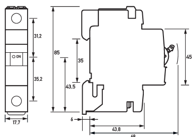
Maßzeichnung Leitungsschutzschalter DLS 6hsl B13-1
