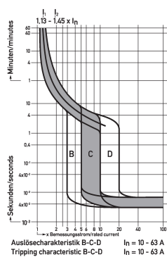
Diagramme Leitungsschutzschalter DLS 6hsl B13-1
