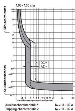
Diagramme Leitungsschutzschalter DLS 6i Z25-3
