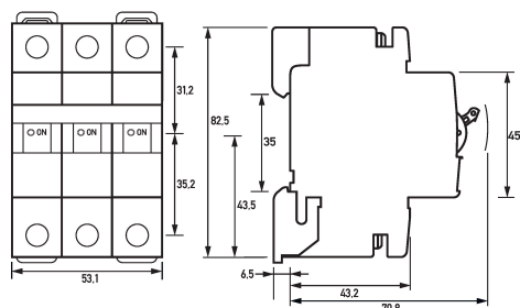
Maßzeichnung Leitungsschutzschalter DLS 6i Z25-3
