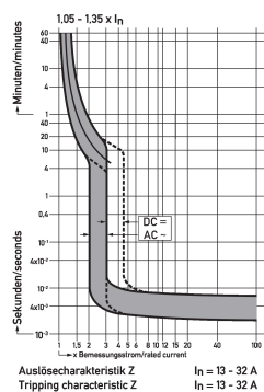
Diagramme Leitungsschutzschalter DLS 6i Z20-3
