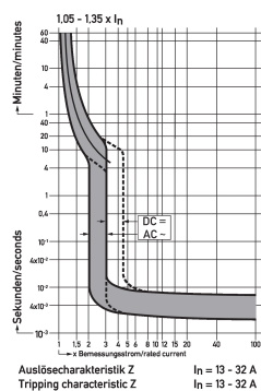
Diagramme Leitungsschutzschalter DLS 6i Z13-3
