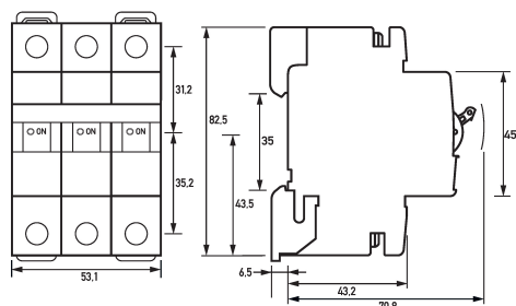
Maßzeichnung Leitungsschutzschalter DLS 6i Z10-3
