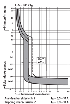
Diagramme Leitungsschutzschalter DLS 6i Z8-3
