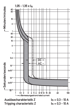
Diagramme Leitungsschutzschalter DLS 6i Z1-3
