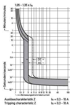
Diagramme Leitungsschutzschalter DLS 6i Zo,8-3
