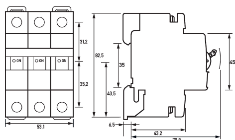
Maßzeichnung Leitungsschutzschalter DLS 6i Zo,8-3
