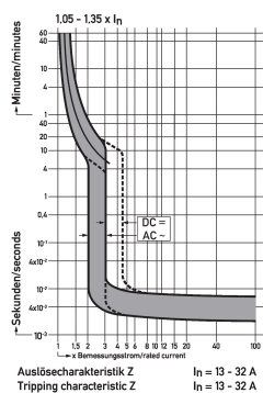
Diagramme Leitungsschutzschalter DLS 6i Z25-2
