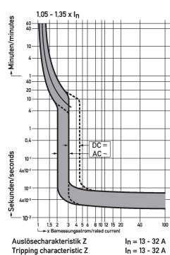
Diagramme Leitungsschutzschalter DLS 6i Z13-2
