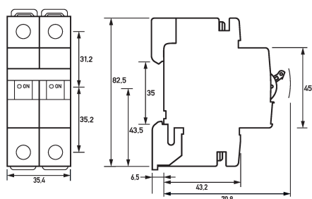
Maßzeichnung Leitungsschutzschalter DLS 6i Z13-2
