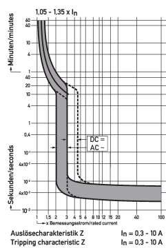
Diagramme Leitungsschutzschalter DLS 6i Z1-2
