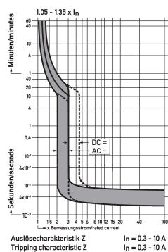
Diagramme Leitungsschutzschalter DLS 6i Zo,3-2
