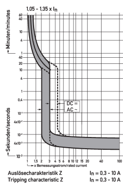
Diagramme Leitungsschutzschalter DLS 6i Zo6-1
