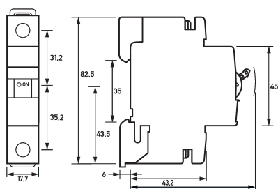
Maßzeichnung Leitungsschutzschalter DLS 6i Zo5-1
