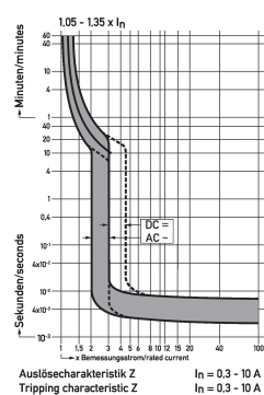
Diagramme Leitungsschutzschalter DLS 6i Zo2-1
