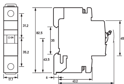
Maßzeichnung Leitungsschutzschalter DLS 6i Zo2-1
