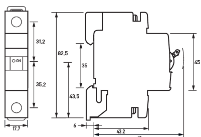
Maßzeichnung Leitungsschutzschalter DLS 6i Zo1-1
