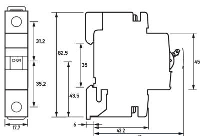
Maßzeichnung Leitungsschutzschalter DLS 6i Zo,3-1
