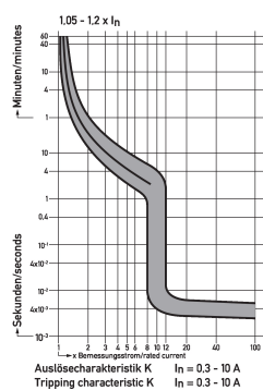
Diagramme Leitungsschutzschalter DLS 6i K 3,5-4
