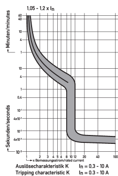
Diagramme Leitungsschutzschalter DLS 6i K2,5-4
