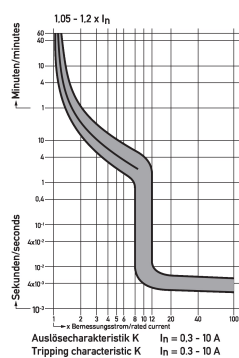
Diagramme Leitungsschutzschalter DLS 6i Ko,3-4
