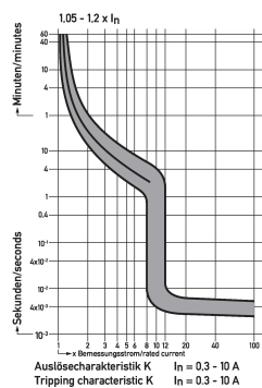
Diagramme Leitungsschutzschalter DLS 6i K5-3+N
