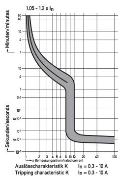
Diagramme Leitungsschutzschalter DLS 6i K 3,5-3+N
