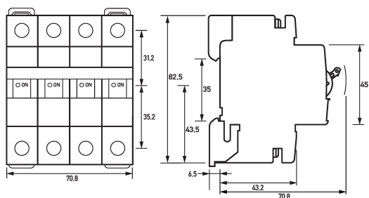
Maßzeichnung Leitungsschutzschalter DLS 6i K 3 -3+N
