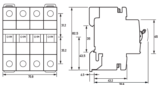
Maßzeichnung Leitungsschutzschalter DLS 6i K2,5-3+N
