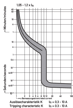
Diagramme Leitungsschutzschalter DLS 6i K2-3+N
