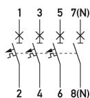
Schaltungsbeispiel Leitungsschutzschalter DLS 6i K2-3+N
