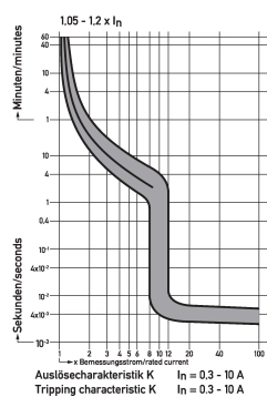
Diagramme Leitungsschutzschalter DLS 6i Ko,8-3+N
