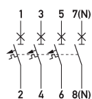
Schaltungsbeispiel Leitungsschutzschalter DLS 6i Ko,8-3+N
