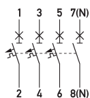
Schaltungsbeispiel Leitungsschutzschalter DLS 6i Ko,5-3+N
