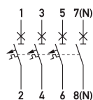
Schaltungsbeispiel Leitungsschutzschalter DLS 6i Ko,3-3+N
