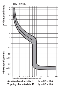
Diagramme Leitungsschutzschalter DLS 6i K5-3
