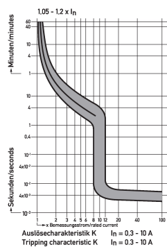
Diagramme Leitungsschutzschalter DLS 6i K1-3
