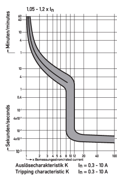
Diagramme Leitungsschutzschalter DLS 6i K 3,5-2
