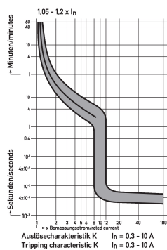
Diagramme Leitungsschutzschalter DLS 6i K1,6-2
