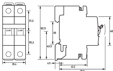
Maßzeichnung Leitungsschutzschalter DLS 6i Ko,8-2
