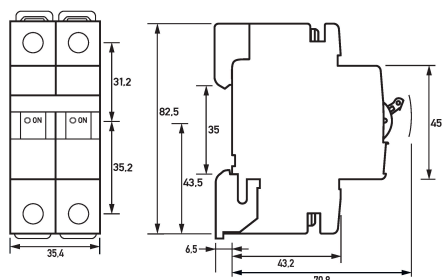
Maßzeichnung Leitungsschutzschalter DLS 6i Ko,8-1+N
