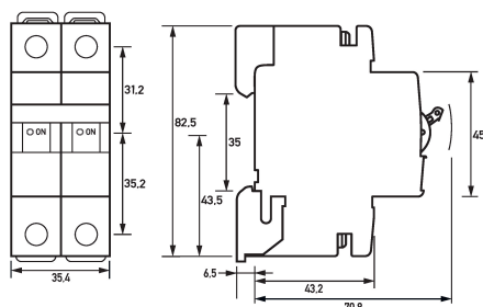
Maßzeichnung Leitungsschutzschalter DLS 6i Ko,5-1+N
