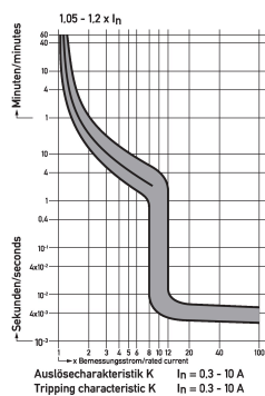
Diagramme Leitungsschutzschalter DLS 6i Ko,5-1+N
