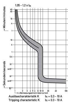
Diagramme Leitungsschutzschalter DLS 6i K 3,5 -1
