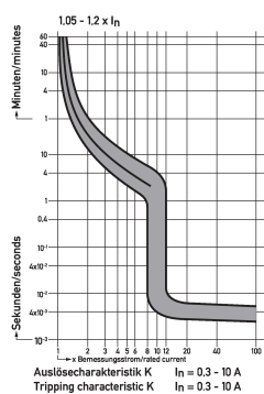
Diagramme Leitungsschutzschalter DLS 6i Ko1-1
