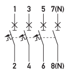
Schaltungsbeispiel Leitungsschutzschalter DLS 6i D5-3+N
