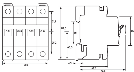
Maßzeichnung Leitungsschutzschalter DLS 6i D4-3+N
