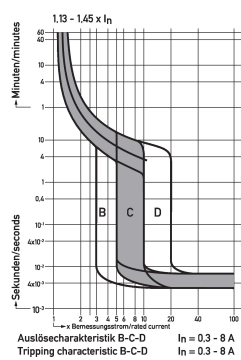
Diagramme Leitungsschutzschalter DLS 6i D4-3+N
