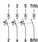
Schaltungsbeispiel Leitungsschutzschalter DLS 6i D1,6-3+N
