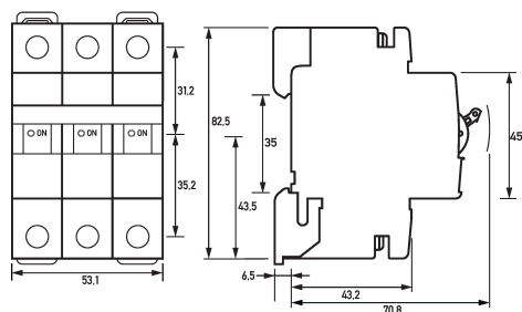
Maßzeichnung Leitungsschutzschalter DLS 6i Do,8-3
