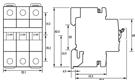
Maßzeichnung Leitungsschutzschalter DLS 6i Do 5-3
