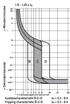
Diagramme Leitungsschutzschalter DLS 6i D 3,5 -2
