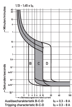
Diagramme Leitungsschutzschalter DLS 6i Do 5-2
