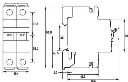
Maßzeichnung Leitungsschutzschalter DLS 6i Do 3-2
