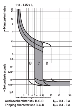
Diagramme Leitungsschutzschalter DLS 6i Do3-1+N
