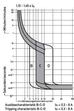
Diagramme Leitungsschutzschalter DLS 6i D1-1+N
