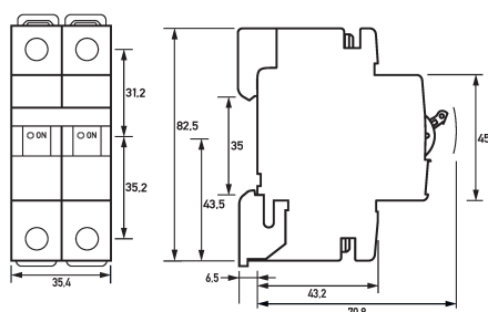
Maßzeichnung Leitungsschutzschalter DLS 6i D1-1+N
