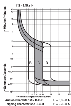
Diagramme Leitungsschutzschalter DLS 6i D03-1
