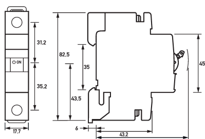
Maßzeichnung Leitungsschutzschalter DLS 6i D2,5-1
